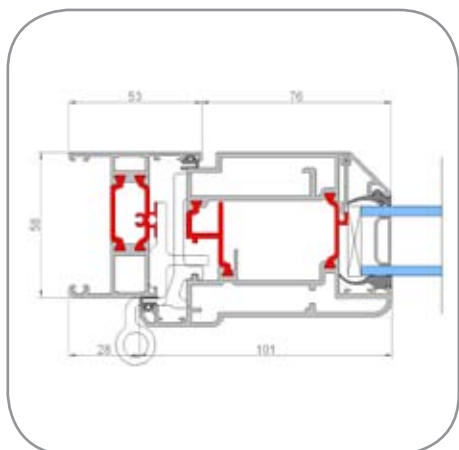
Jamb Detail
